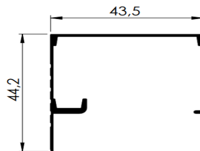
BX 403 Caixa superior nova
