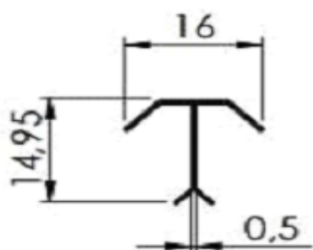
DS0002 Cantoneira sextavada
