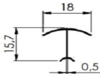
DS0003 Cantoneira boleada
