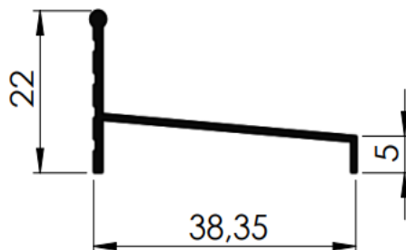
BX 404 Trilho inferior novo
